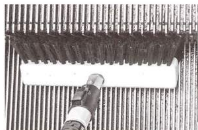
写真2 3つの面からできているブラシ。③は湾曲した溝の底に届くようになっている
